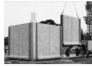
1972-1983. Centre de calcul scientifique de l'armement (CCSA), CELAR, Bruz (Ille-et-Vilaine) : vue de la pose d'éléments préfabriqués sur le chantier, 29 oct. 1973 (cliché anonyme). (Dossier 112 Ifa 1500/36. Doc. NR-10-12-09-06)
